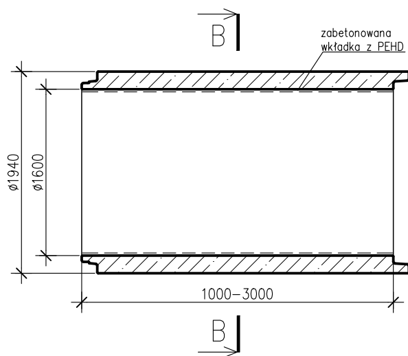
PRZEKRÓJ B-B
